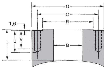
MONTAGGIO SUL MANTELLO SHELL MOUNT
