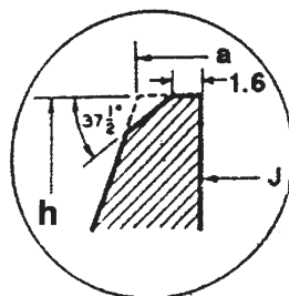
Dettaglio smusso Bevel detail
